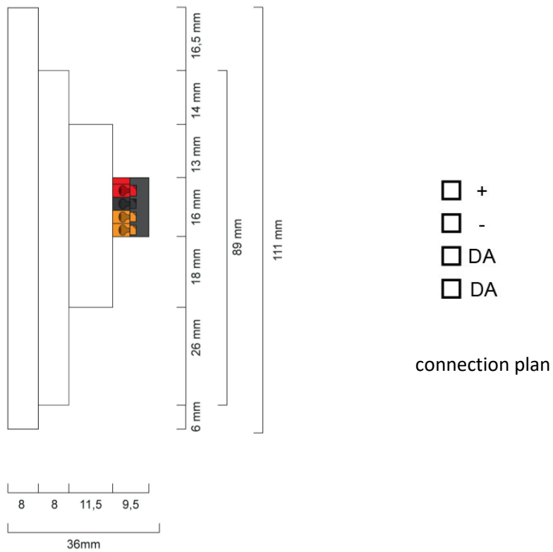
dimensions Art.Nr.: 86456840-...
