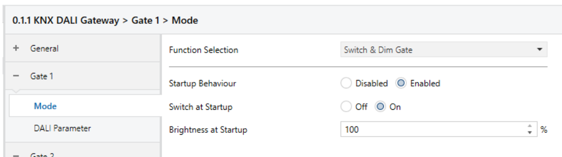
Fig.13 Gate Settings ETS: Tab „Mode“ Switch & Dim Gate
